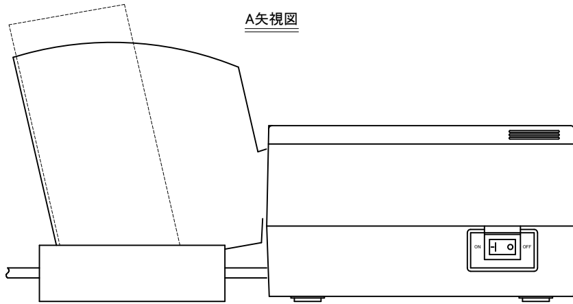
B矢视图
